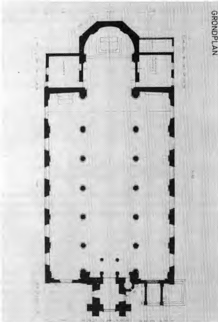
47. Grondplan van de kerk (reproductie J. De Coninck, 1968)
